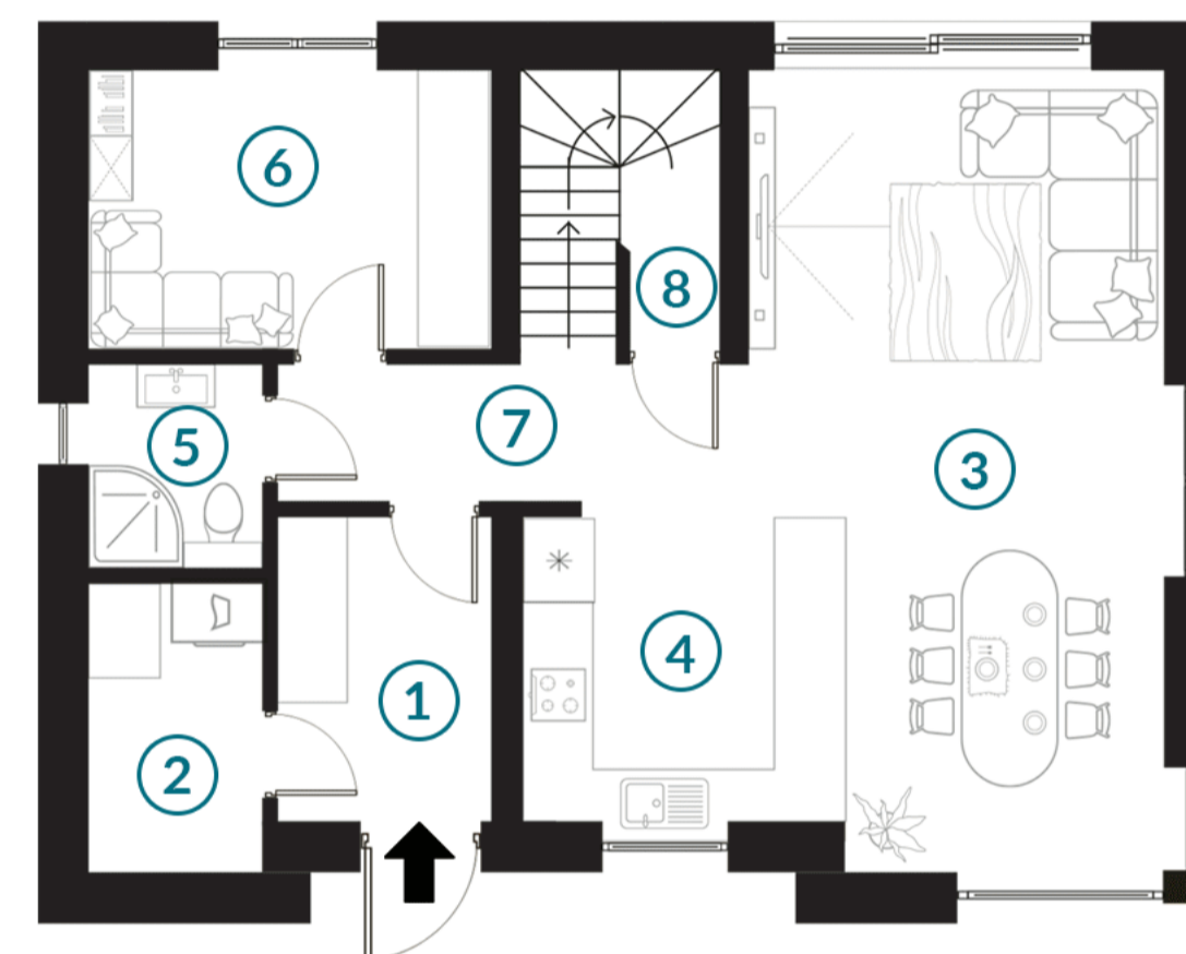
RZUT PARTERU
